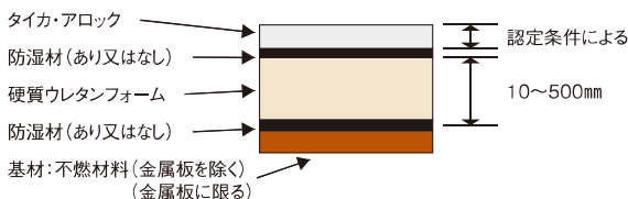
構造説明図
